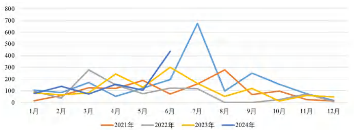
图 5—3 鄂城区新港（闸下）雨量站月降雨量曲线变化图
