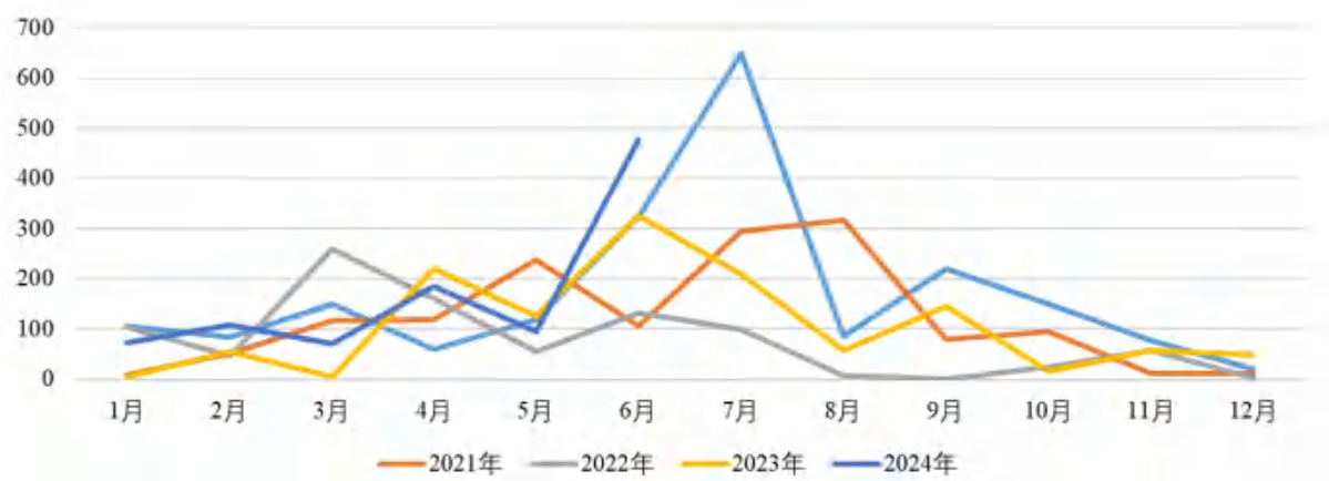
图 5-1 华容区红莲湖雨量站月降雨量曲线变化图
